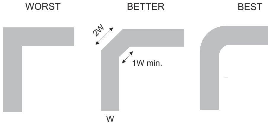
图 10-1. 布线示例
