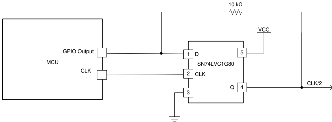
图 8-1. 时钟分频
