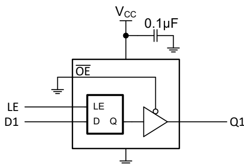
图 8-1. 典型应用框图
