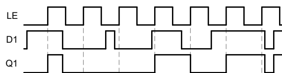
图 8-2. 应用时序图
