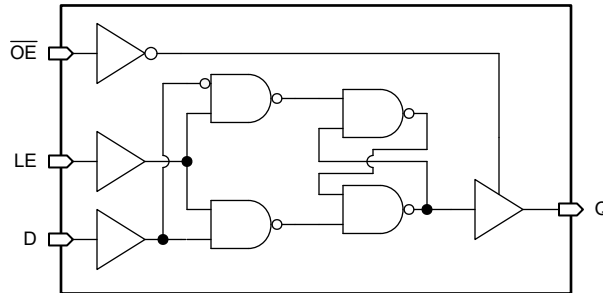
功能方框图
