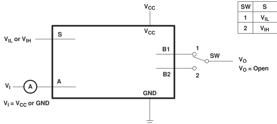
图 6-3. 导通状态开关漏电流测试电路
