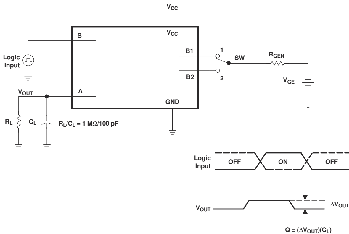
图 6-8. 电荷注入测试
