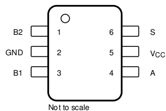
图 4-2. DCK 封装 6 引脚 SC70 顶视图
