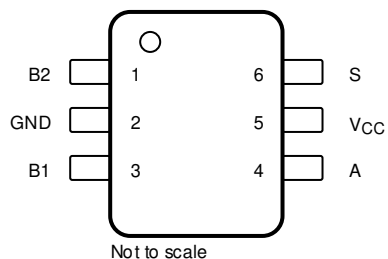
图 4-1. DBV 封装 6 引脚 SOT-23 顶视图
