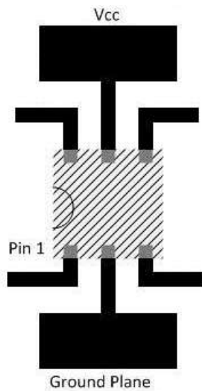
图 10-1. 推荐布局示例
