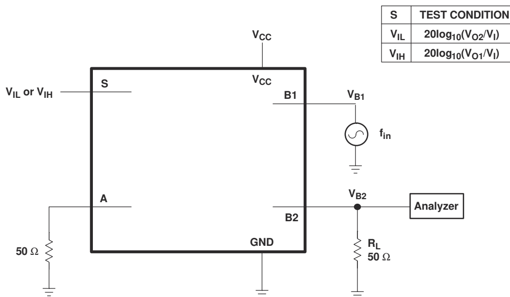
图 6-6. 串扰 ( 开关间 )
