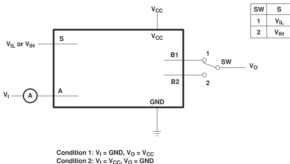
图 6-2. 关断状态开关漏电流测试电路
