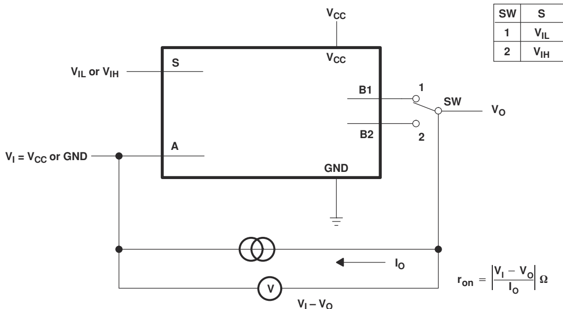
图 6-1. 导通电阻测试电路
