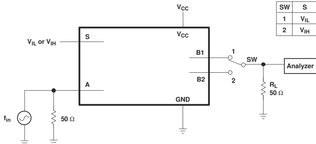
图 6-7. 馈通
