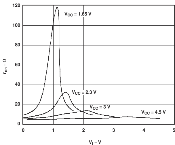
图 5-1. 典型 R_{on} 与输入电压 ( V_I ) 之间的函数关系 ( V_I = 0 至 V_{CC} )
