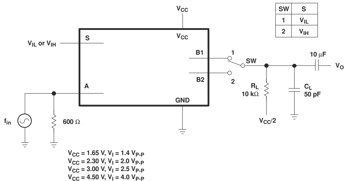
图 6-9. 总谐波失真
