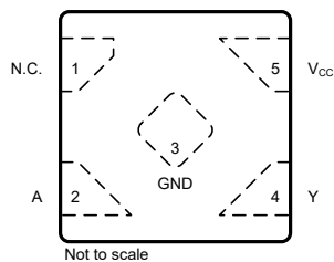
图 4-2. DTX 封装 5 引脚 X2SON 顶视图
