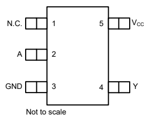
图 4-1. DCK、DBV 封装 5 引脚 SC70、SOT-23 顶视图
