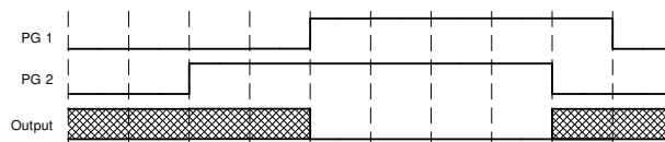
图 8-2. 典型应用时序图
