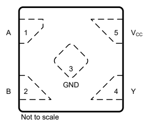
图 4-2. DTX 封装 5 引脚 X2SON 顶视图
