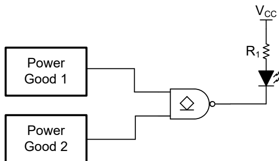
图 8-1. 典型应用框图
