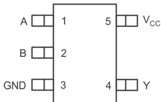
图 4-1. DCK、DBV 封装 5 引脚 SC70、SOT-23 顶视图
