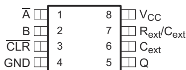
图 4-2. DCU 封装 8 引脚 VSSOP 顶视图
