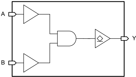
逻辑图
