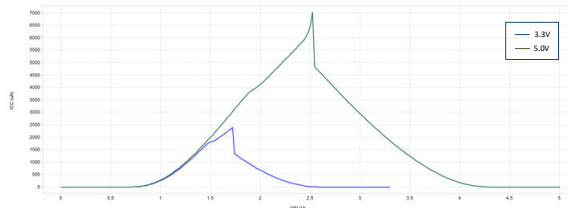
图 5-2. 电源电流与输入电源电压 (3.3V 至 5.0V) 间的关系
