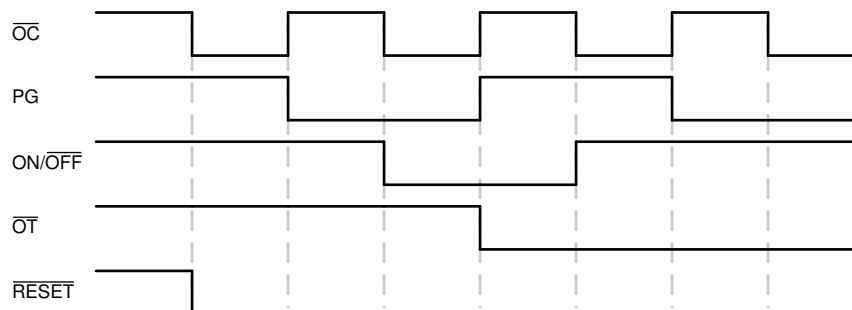
图 8-2. 应用时序图
