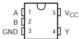
图 4-1. DCK 封装, 5 引脚 SOT-SC70 (顶视图)
