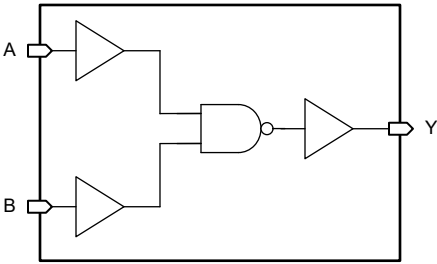
逻辑图
