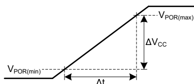
图 8-1. 已知上电状态的电源 (V CC ) 斜坡特性
