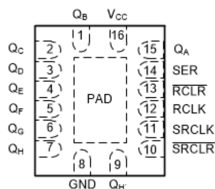
图 4-2. BQB 封装，16 引脚 WQFN ( 透明顶视图 )
