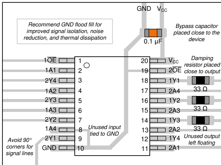
图 10-3. SN74LV8T244-EP 采用 TSSOP 封装的示例布局
