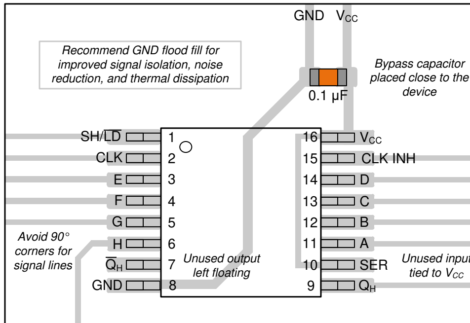
图 8-3. 采用 TSSOP 封装的 SN74LV8T165 的示例布局
