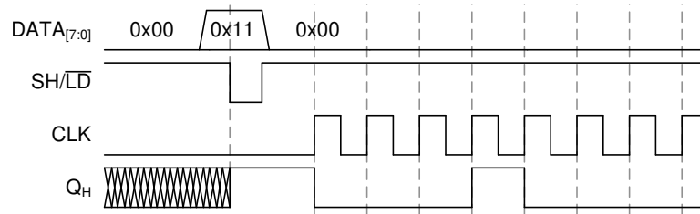
图 8-2. 应用时序图
