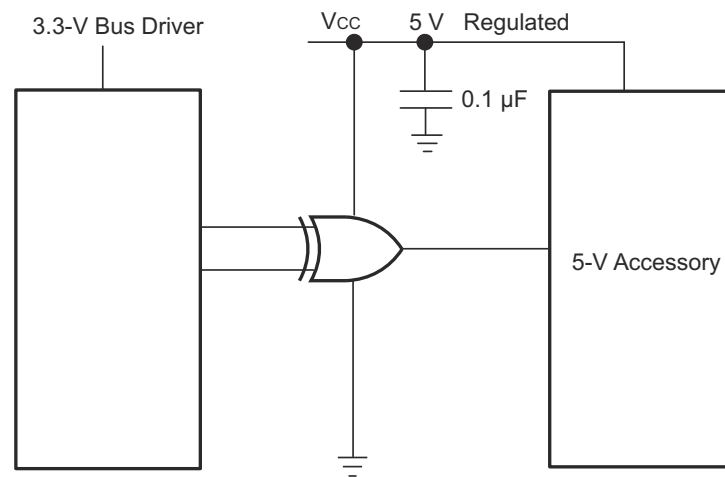
图 8-1. 典型应用原理图
