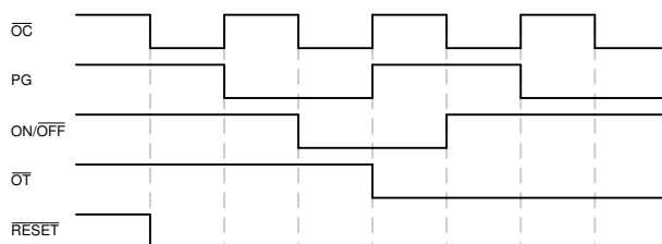
图 9-2. 应用时序图
