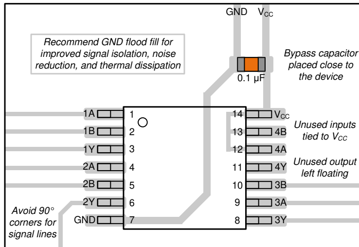
图 11-1. 示例布局 SN74LV4T08
