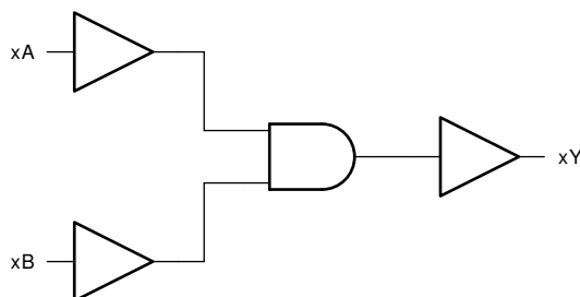
简化逻辑图 (正逻辑)
