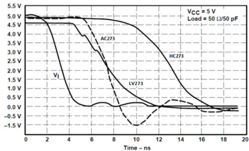
图 9-2. 开关特性比较
