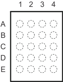
图 5-3. GQN 或 ZQN 封装，20 引脚 BGA ( 顶视图 )
