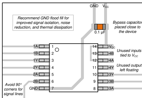
图 8-3. SN74HCS7266-Q1 的示例布局
