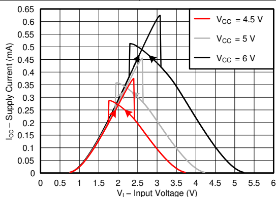
图 5-3. 不同常见电源电压值下 (4.5V 至 6V) 下典型电源电流与输入电压间的关系
