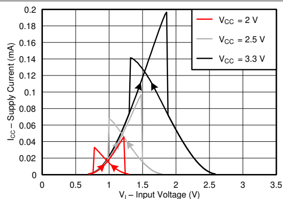
图 5-2. 不同常见电源电压值下 (2V 至 3.3V) 下典型电源电流与输入电压间的关系
