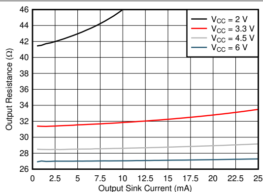
图 5-1. 低电平状态下的输出驱动器电阻
