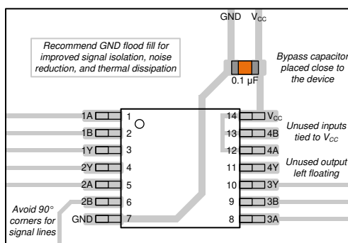
图 8-3. SN74HCS266 的示例布局
