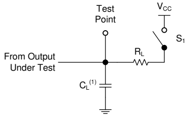
图 6-1. 负载电路
