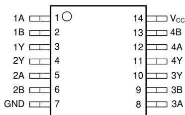
图 4-1. PW 或 D 封装 14 引脚 TSSOP 或 SOIC 顶视图
