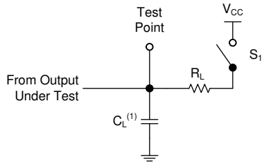
图 6-1. 负载电路
