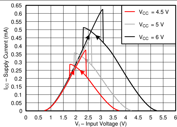
图 5-3. 常见电源值 (4.5V 至 6V) 下典型电源电流与输入电压间的关系
