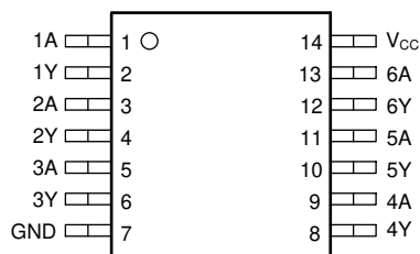
图 4-1. PW、D 或 DYY 封装；14 引脚 TSSOP、SOIC 或 SOT-23 顶视图
