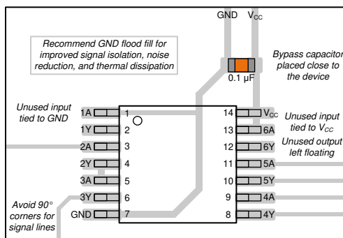
图 8-3. SN74HCS05 的示例布局
