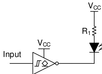
图 8-1. 典型应用框图
