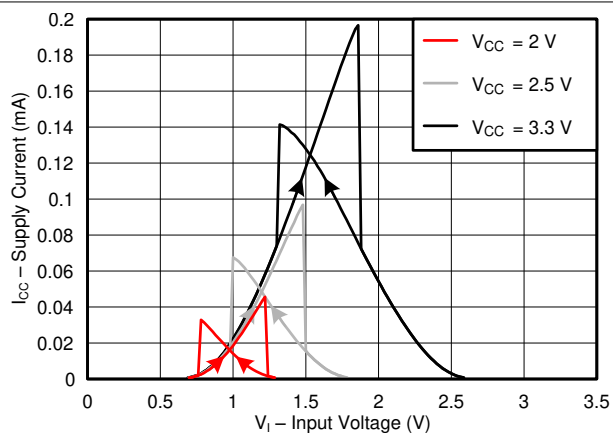
图 5-2. 常见电源值 (2V 至 3.3V) 下典型电源电流与输入电压间的关系
