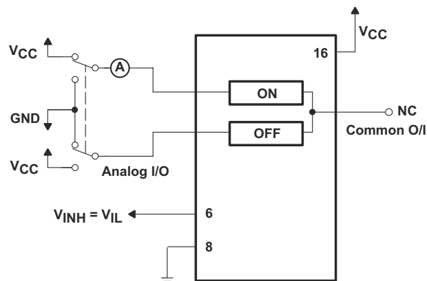
图 6-4. 开启通道最大漏电流，通道间，测试设置
