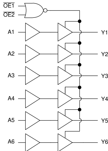
功能方框图
