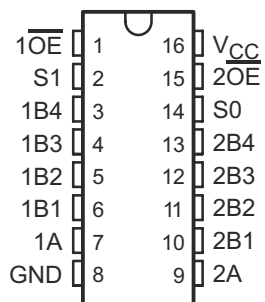
图 4-1. PW 或 DYY 封装 16 引脚 TSSOP 或 SOT 顶视图
