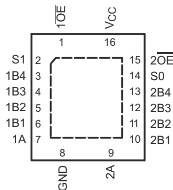
图 4-2. BQB 封装 16 引脚 VQFN 顶视图
