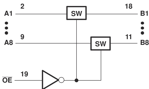
图 7-1. 逻辑图 (正逻辑)
