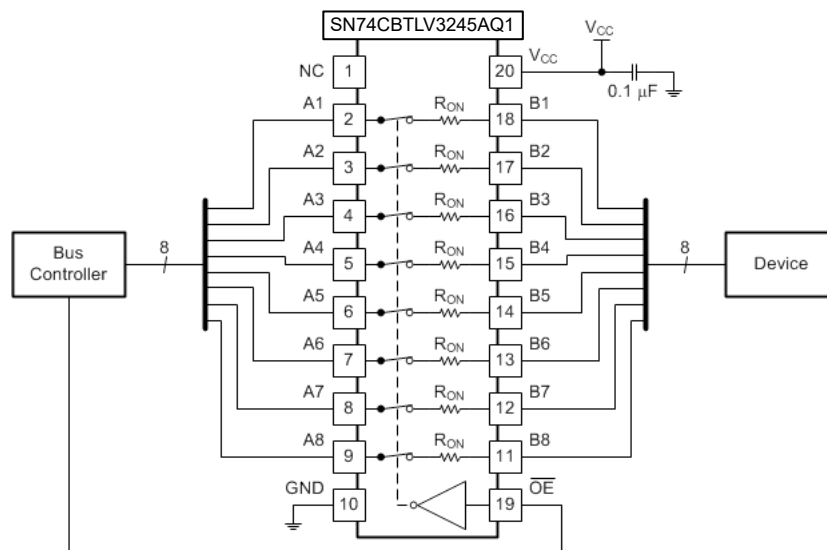
图 8-1. 典型应用原理图
