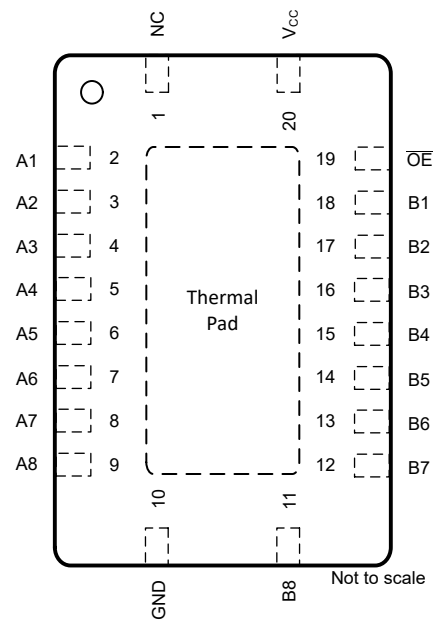
图 4-2. RKS 封装 20 引脚 VQFN (顶视图)
