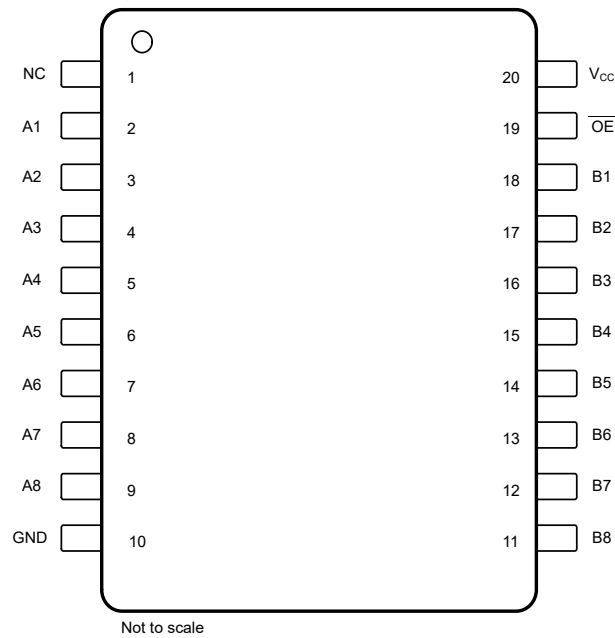
图 4-1. DGS、PW 封装 20 引脚 VSSOP 和 TSSOP (顶视图)
