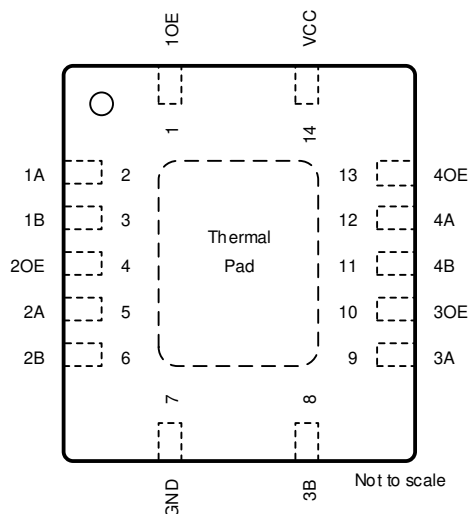
图 4-2. BQA 封装，14 引脚 WQFN (顶视图)
