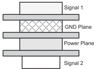
图 8-3. 示例布局
