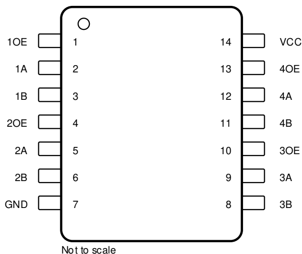
图 4-1. PW 和 DYY 封装，14 引脚 TSSOP 和 SOT (顶视图)
