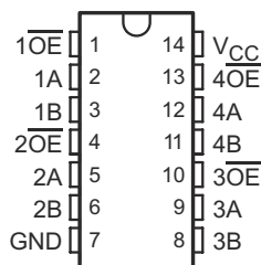
图 4-1. PW、DYY 封装 14 引脚 TSSOP、SOT 顶视图
