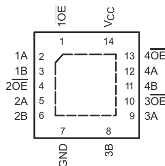
图 4-2. BQA 封装 14 引脚 WQFN 顶视图
