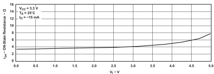
图 4-1. 典型的 r_{on} 与 V_I 间的关系
