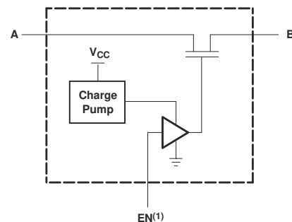
每个 FET 开关 (SW) 的简化版原理图
