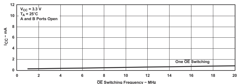
图 4-2. 典型的 I_{CC} 与 \overline{OE} 开关频率间的关系
