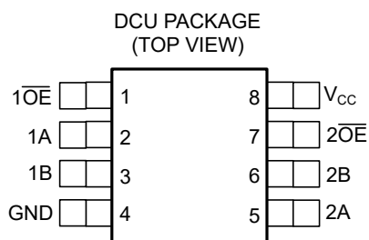
图 3-1. DCU 封装 8 引脚 (俯视图)
