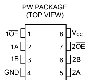
图 3-2. PW 封装 8 引脚 (俯视图)
