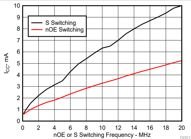
图 4-2. 典型 I_{CC} 与 \overline{OE} 开关频率间的关系, V_{CC} = 3.3V
