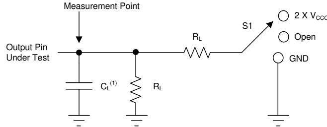
图 6-1. 负载电路
