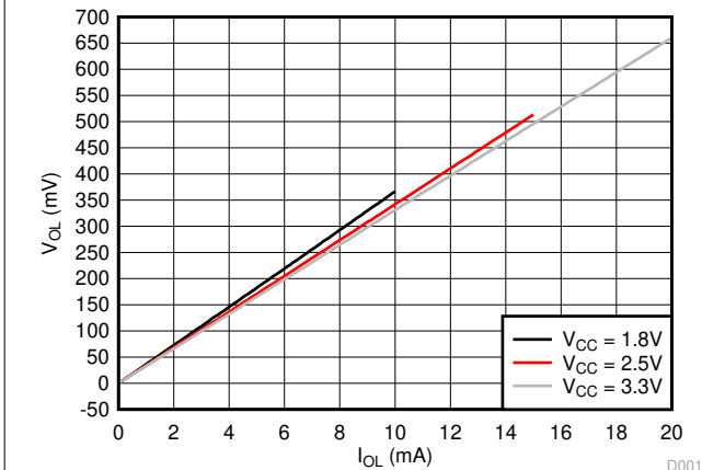
图 5-3. 典型 ( T_A=25^\circ\text{C} ) 输出低电压 ( V_{OL} ) 与灌电流 ( I_{OL} ) 间的关系
