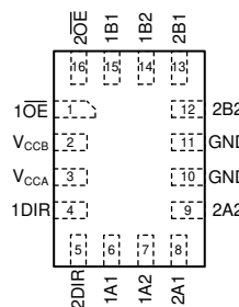
图 4-3. RSV 封装，16 引脚 UQFN（透明顶视图）
