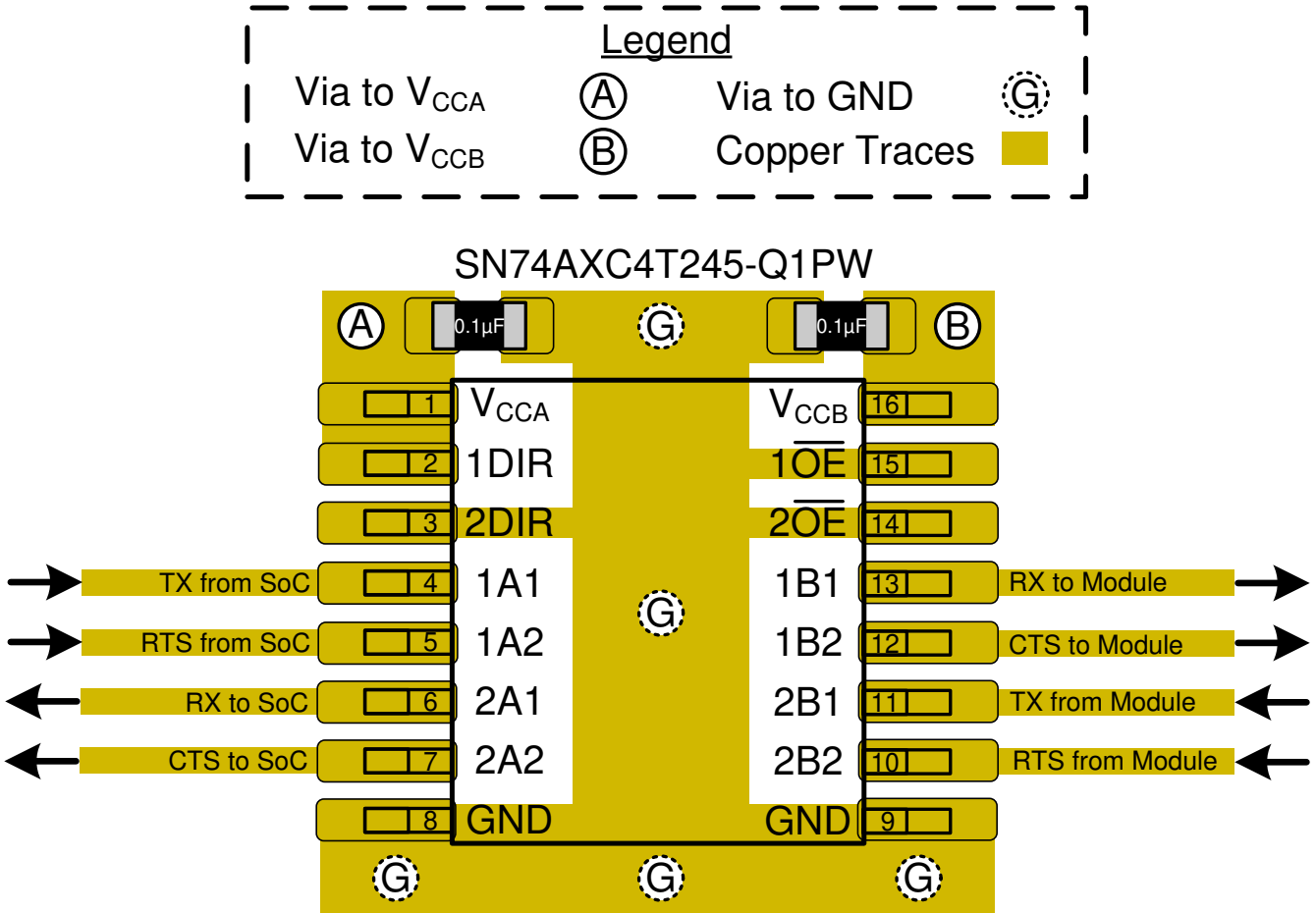
图 8-3. 布局示例
