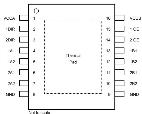
图 4-4. DYY 封装, 16 引脚 SOT (顶视图)
