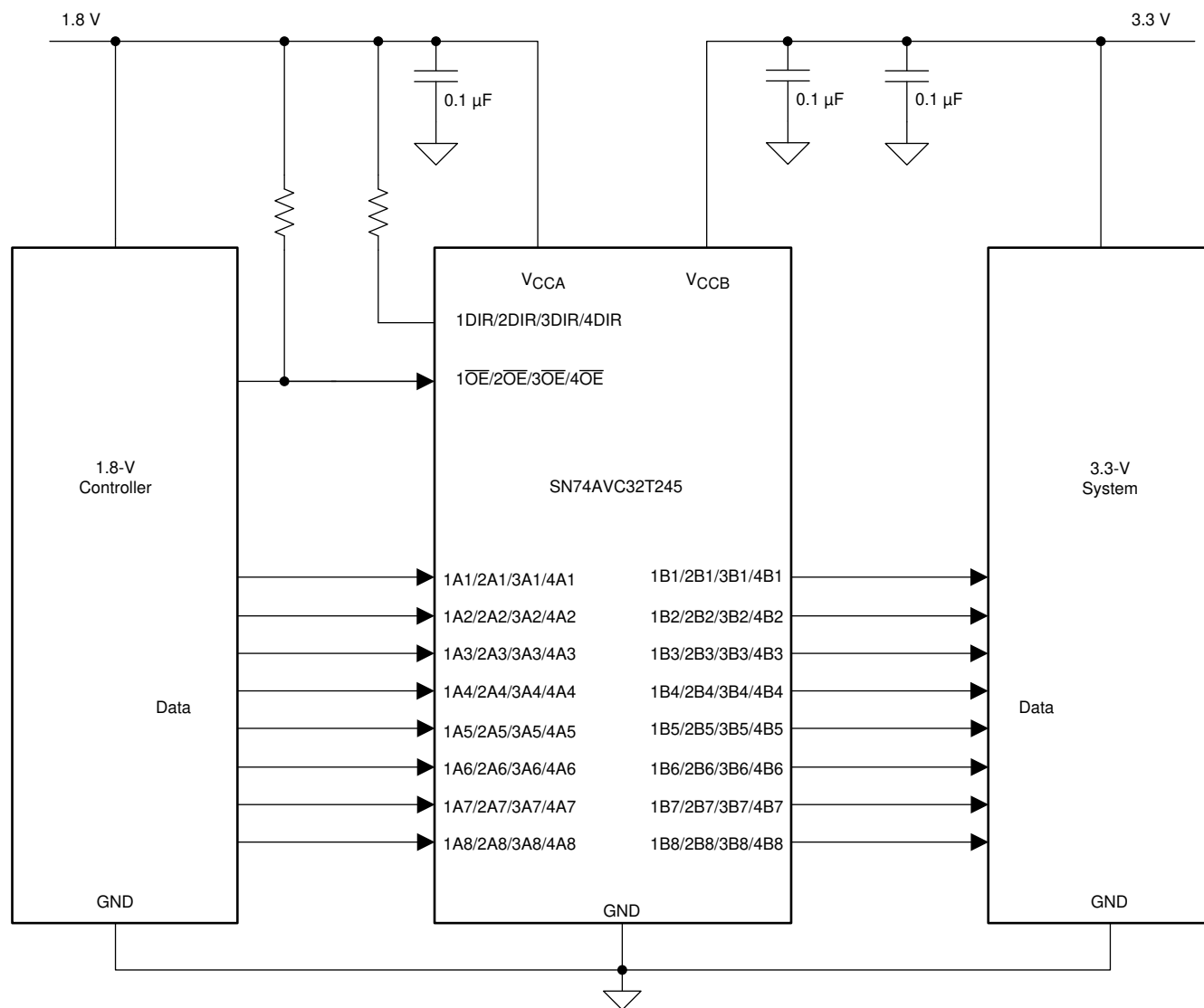
图 10-1. 应用原理图
