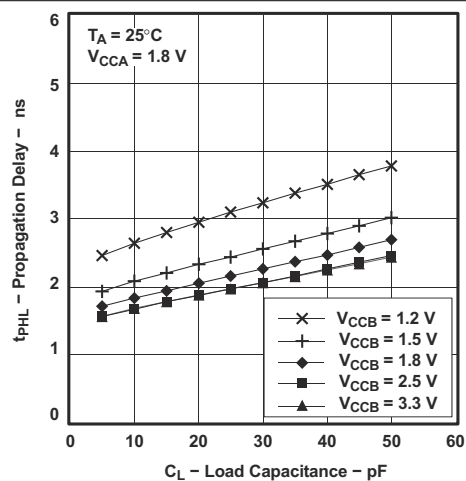
图 7-6. 典型传播延迟 t_{PLH} (A 到 B) 与负载电容间的关系
