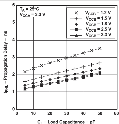
图 7-10. 传播延迟与负载电容间的关系
