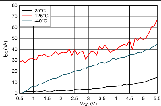
图 5-2. 电源电压两端的电源电流
