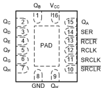
图 4-2. WBQB 封装， 16 引脚 WQFN (透明顶视图)
