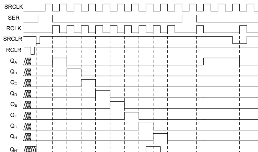
图 5-1. 时序图
