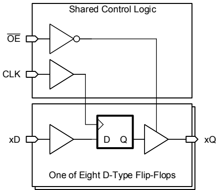
功能方框图
