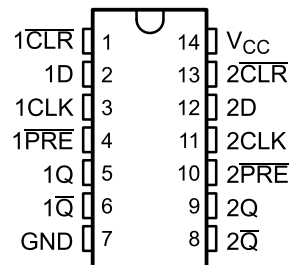
图 4-2. SN74AHC74 D、DB、DGV、N、NS 或 PW 封装，14 引脚 SOIC、SSOP、TVSOP、PDIP、SO 或 TSSOP（顶视图）
