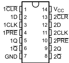
图 4-1. SN54AHC74 J 或 W 封装，14 引脚 CDIP 或 CFP（顶视图）
