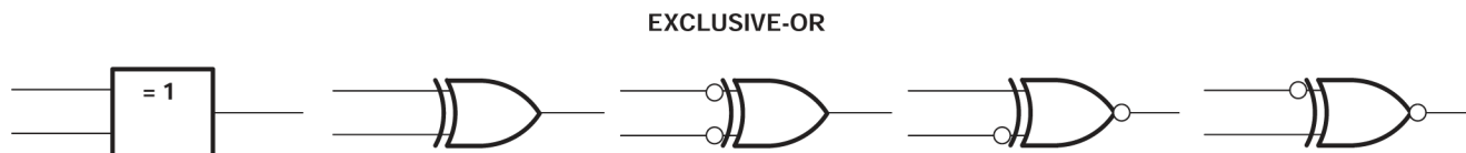
图 6-1. 异或逻辑
