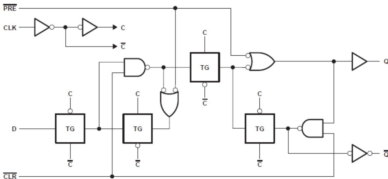
逻辑图 ( 正逻辑 )
