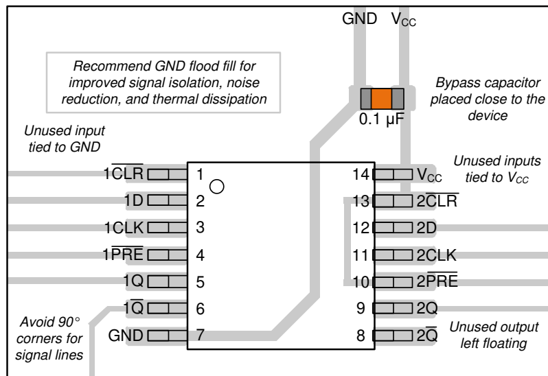
图 7-1. SNx4ACT74 封装的示例布局
