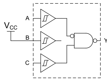
具有 1 个反相输入的双输入与非门
