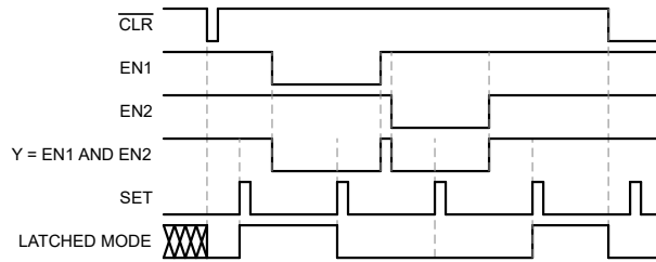
图 8-2. 典型应用时序图
