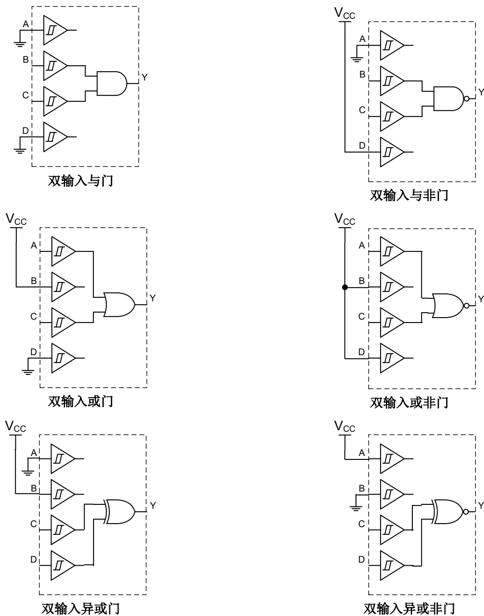
图 7-2. 逻辑配置
