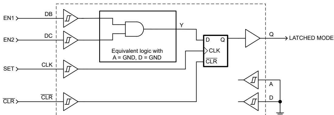
图 8-1. 典型应用原理图
