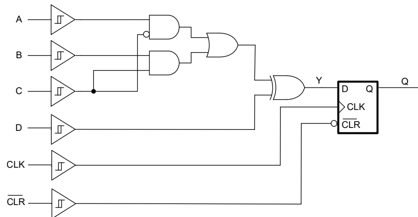
逻辑图（正逻辑）
