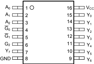
PW 封装，16 引脚 TSSOP（顶视图）
