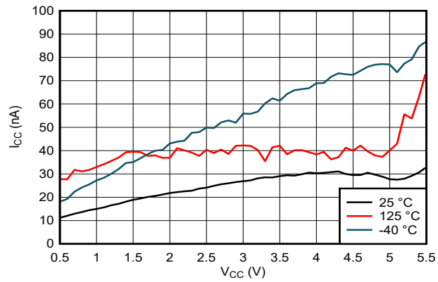
图 5-2. 电源电流与电源电压的关系
