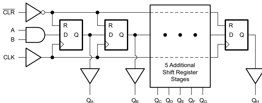
图 7-1. SN74ACT164-Q1 的逻辑图 (正逻辑)
