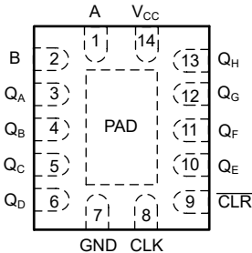
图 4-2. WBQA 封装 14 引脚 WQFN (顶视图)
