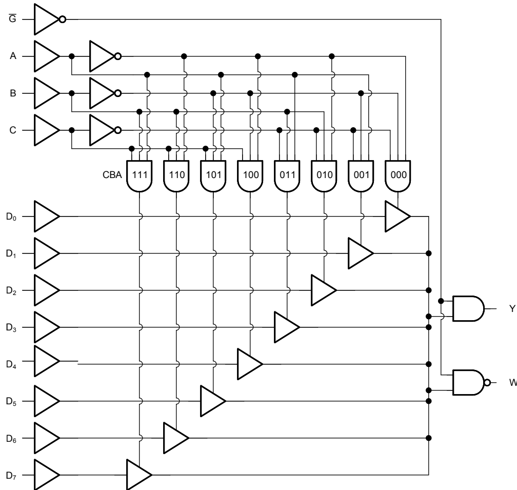
图 7-1. SN74ACT151-Q1 的逻辑图 (正逻辑)
