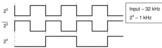
图 8-2. 应用时序图
