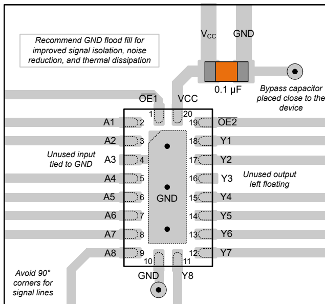
图 8-3. 采用 RKS 封装的 SN74AC541-Q1 的示例布局
