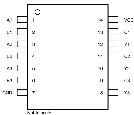
图 4-1. SN74AC3G97 PW 封装，14 引脚 TSSOP ( 顶视图 ) 图 4-2. SN74AC3G97 BQA 封装，14 引脚 WQFN ( 顶视图 )
