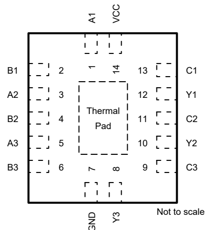
图 4-1. SN74AC3G97 PW 封装，14 引脚 TSSOP ( 顶视图 ) 图 4-2. SN74AC3G97 BQA 封装，14 引脚 WQFN ( 顶视图 )
