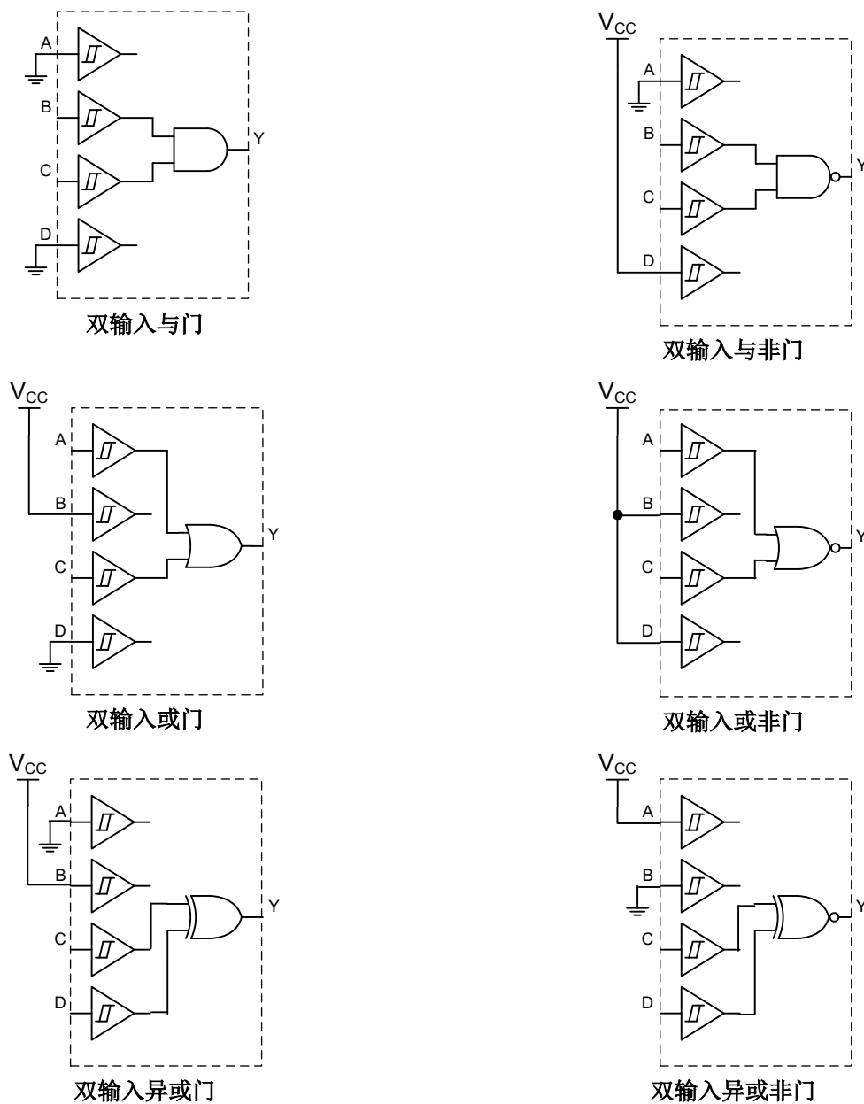
图 7-3. 逻辑配置
