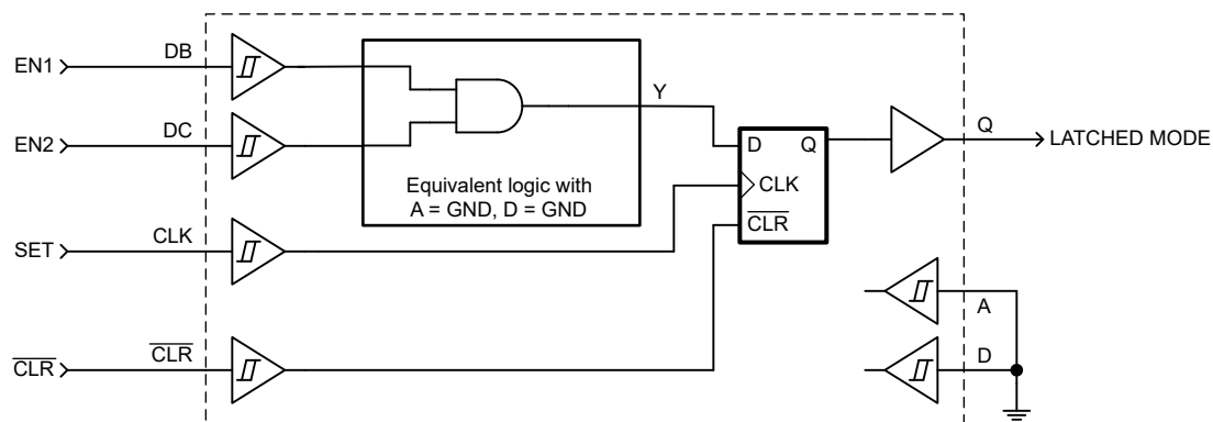
图 8-1. 典型应用原理图
