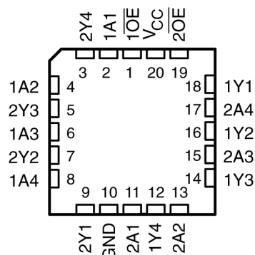
图 4-2. SN54AC240 FK Package (Top View)
