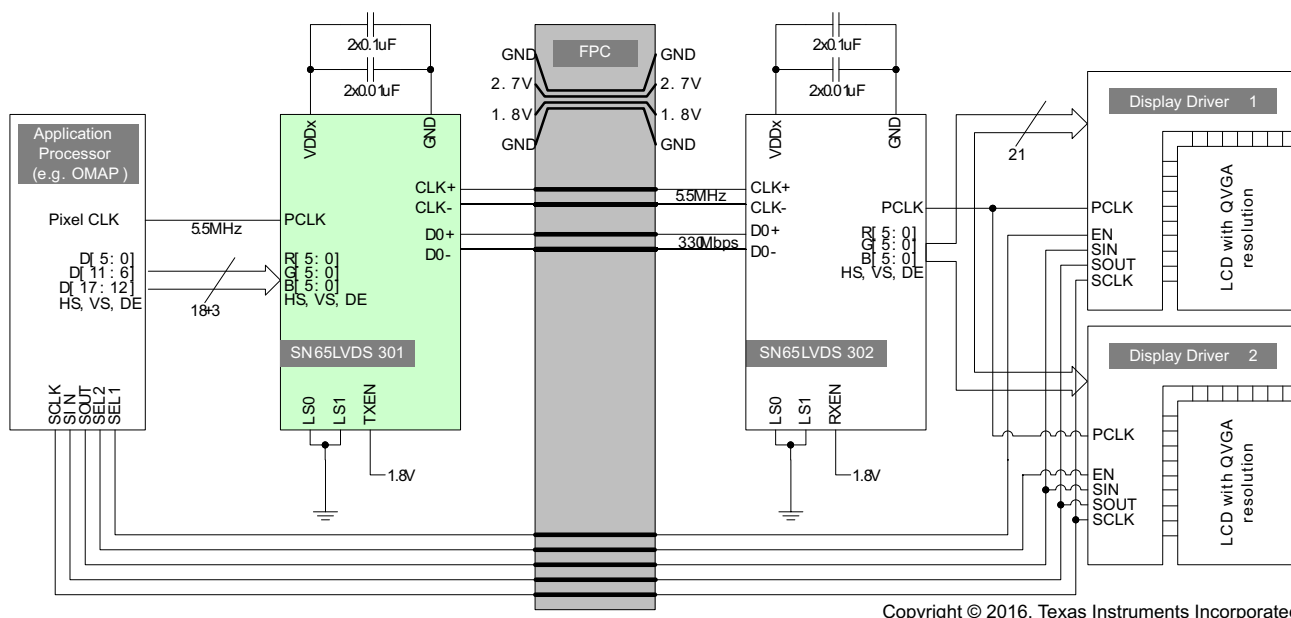
图 9-9. Example Dual-QVGA Display Application
