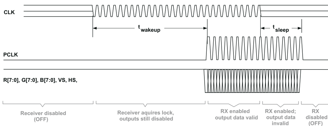
图 7-11. Standby Detection
