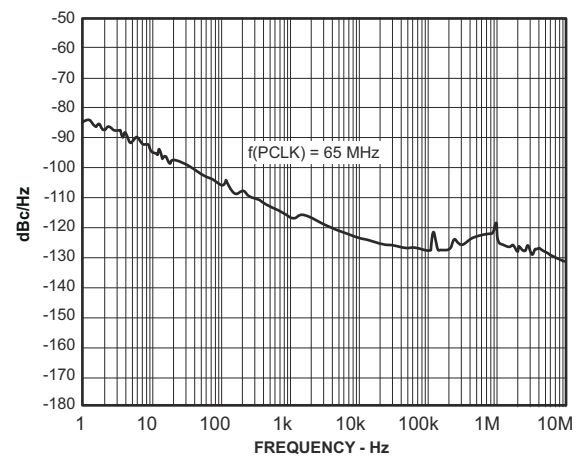
图 6-17. Phase Noise
