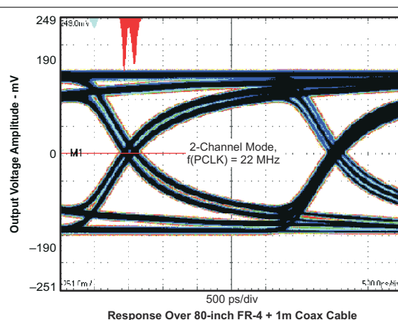
图 9-7. VGA 2-Channel Output Waveform
