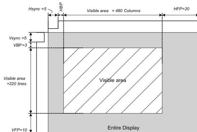
图 9-1. HVGA Display
