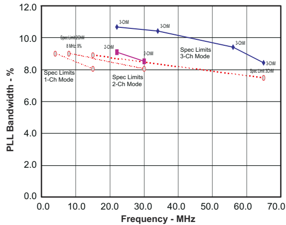
图 6-7. PLL Bandwidth
