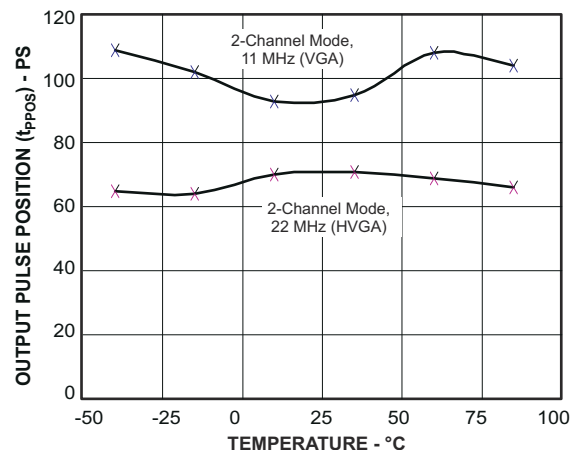
图 6-9. Output Pulse Position vs Temperature
