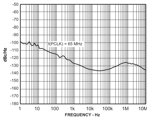
图 6-18. PLL Phase Noise
