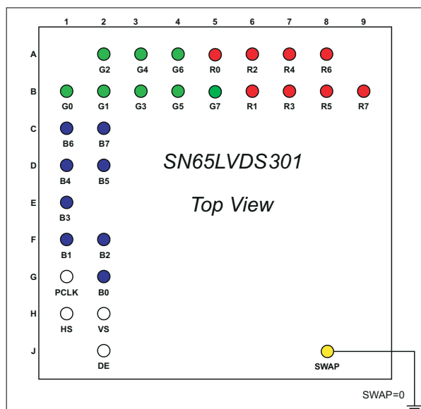
图 8-2. SWAP PIN = 0
