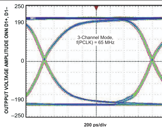
图 6-11. Data Eye Pattern, 3-channel Mode
