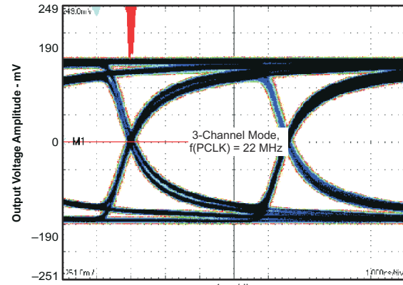
图 6-15. VGA 3-channel Output Waveform
