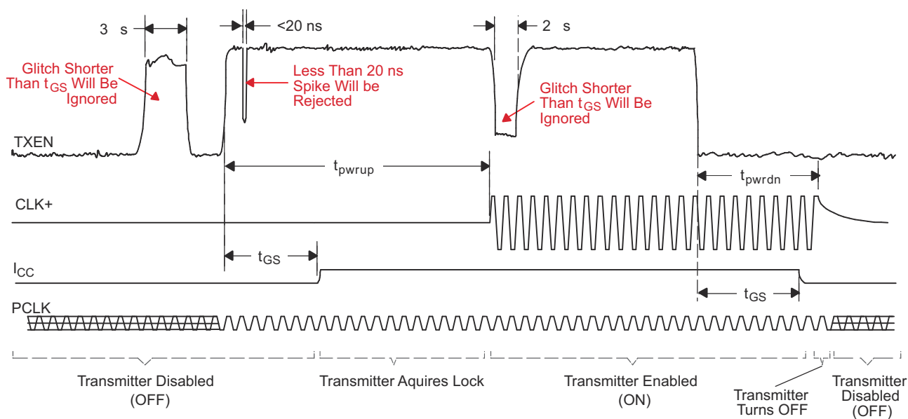
图 7-8. Transmitter Enable Glitch Suppression Time
