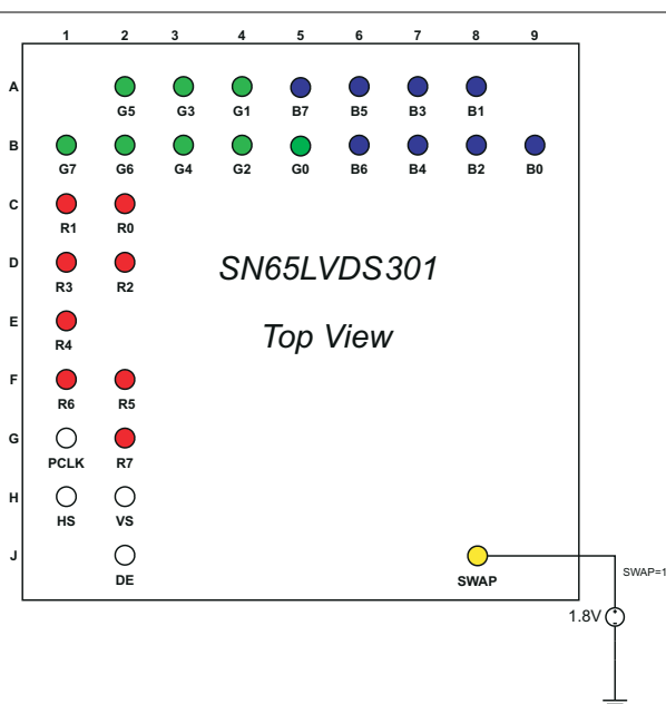
图 8-3. SWAP PIN = 1
