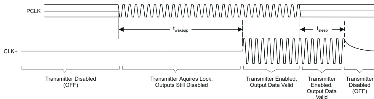
图 7-9. Standby Detection
