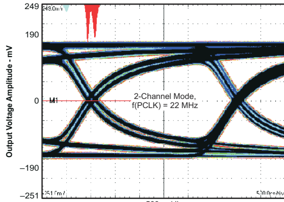
图 6-14. VGA 2-channel Output Waveform
