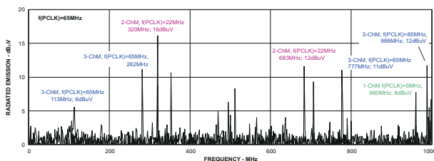
图 6-22. GTEM SAE J1752/3 EMI Test
