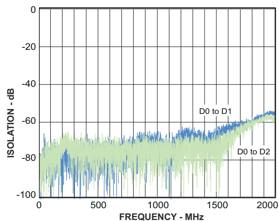
图 6-21. Crosstalk
