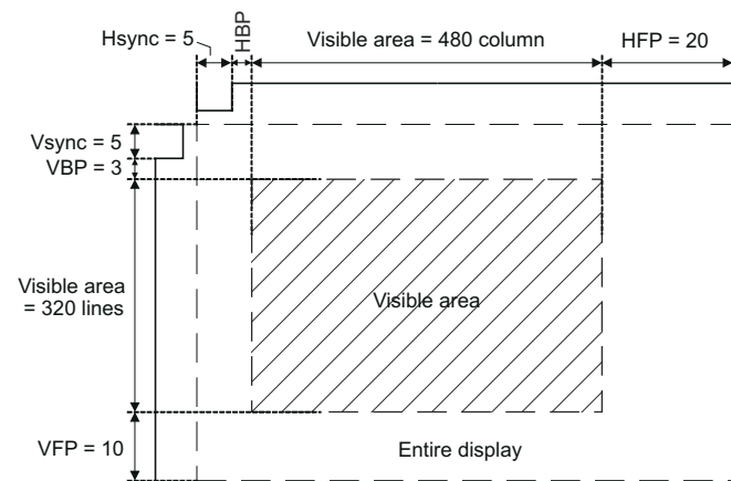
图 9-3. HVGA Display Parameters
