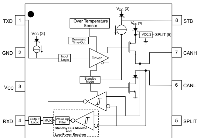
方框图
